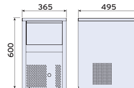
CIM 20/5
